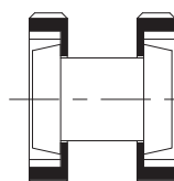
Riduzioni DIN M a DIN M Reducer NUT-NUT
